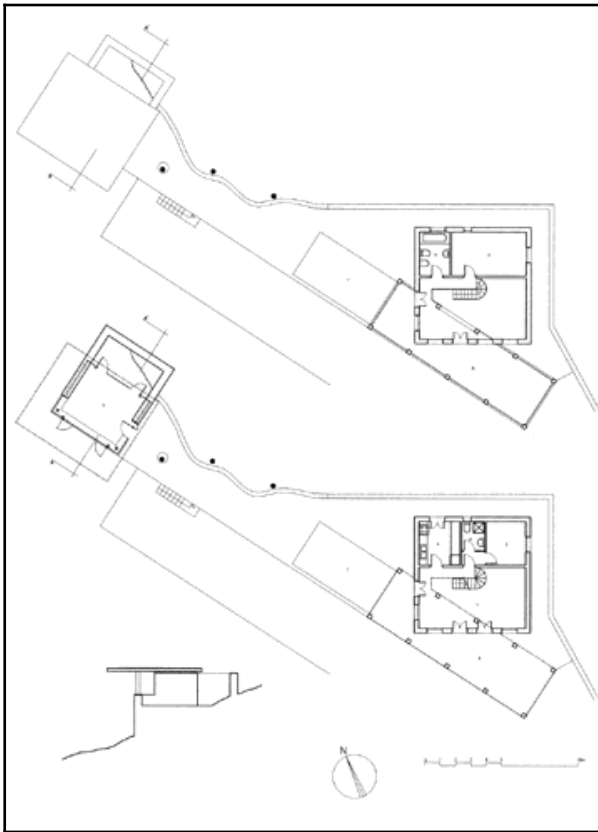
plantas generales y sección general plan and section
