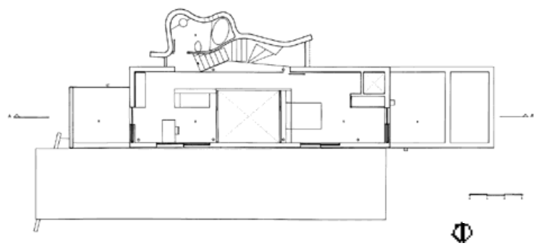
planta primera first floor
