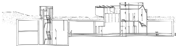
sección transversal 2 cross section 2
