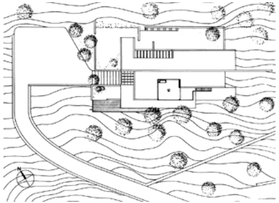
planta de situación site plan
