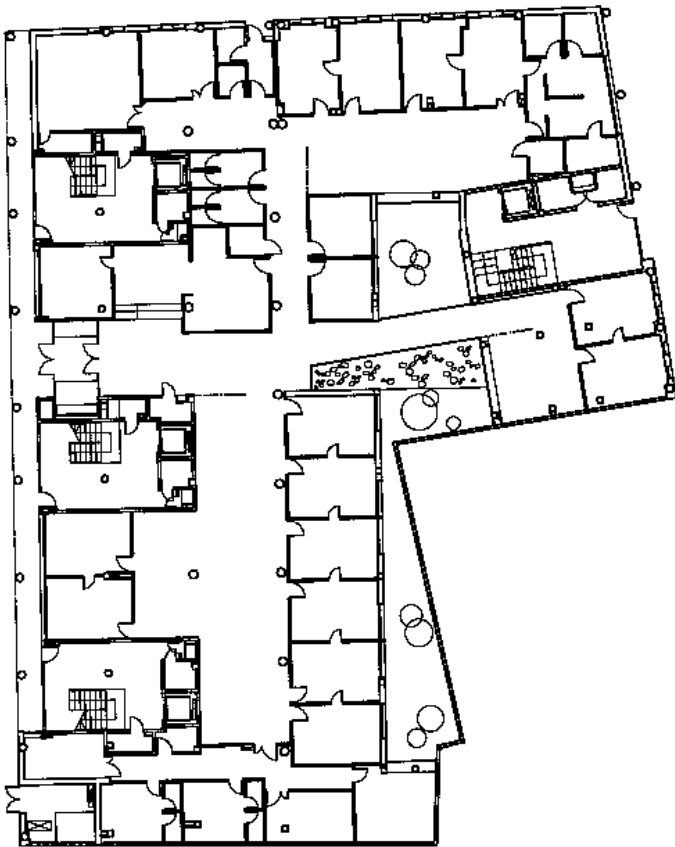
planta baja con el centro de asistencia primaria ground floor plan with the primary health centre
